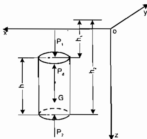
Hình 2-23. Sơ đồ minh họa định luật Acsimet
