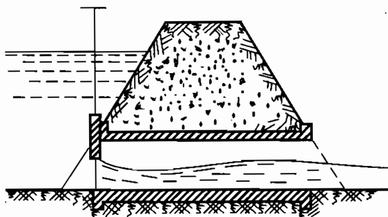
Hình 9-4. Dòng chảy qua cống ngầm
