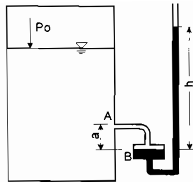
Hình 2-15. Áp kế thủy ngân kiểu chậu
