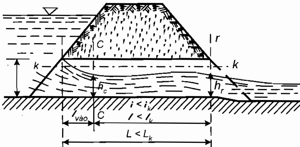
Hình 9-12. Trường hợp 0 < i < i_p .
