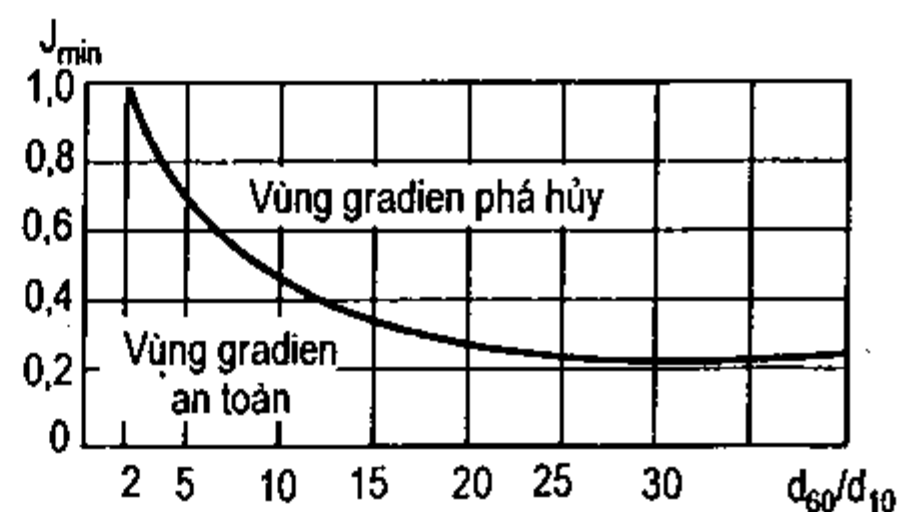
Hình VIII-22. Đồ thị quan hệ giữa gradien thấm tối thiểu (an toàn) và mức độ không đồng nhất của đất khi dòng thấm từ dưới đi lên.
