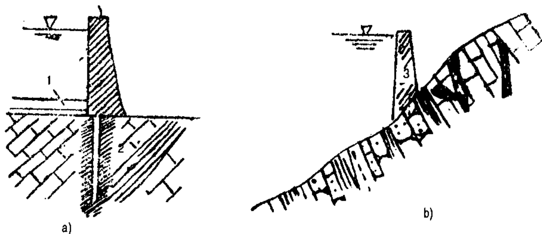
Hình VIII-25. Xử lý karst.
