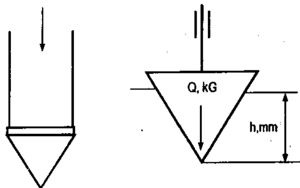
Hình V-14. Sơ đồ mũi xuyên tĩnh
