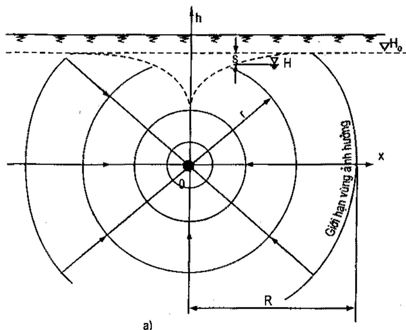
Hình VII-15. Mô hình dòng thấm tới giếng đơn không hoàn chỉnh.
