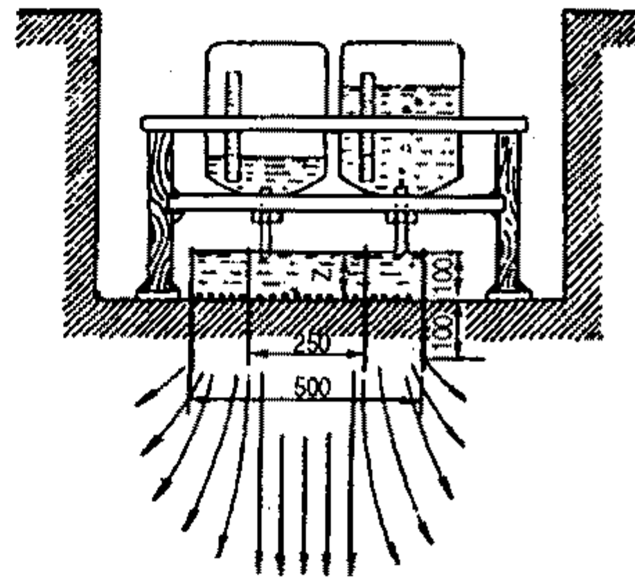
Hình IX-8. Phương pháp thí nghiệm của Nectarov
