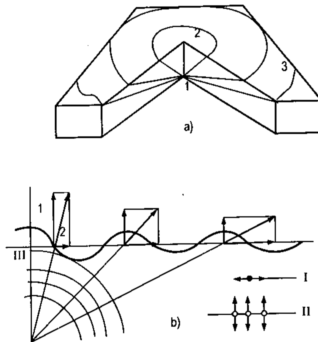
Hình VIII-39. Sơ đồ truyền sóng động đất
