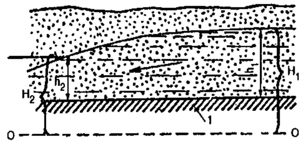
Hình VI-1. Sơ đồ một tầng chứa nước theo mặt cắt đứng dọc theo đường dòng 1. 1. Đáy cách nước (tường) ; 2. Mặt thoáng tự do (mái); h_1 , H_1 và h_2 , H_2 - Chiều dày và áp lực dòng thấm tại tiết diện 1 và 2.
