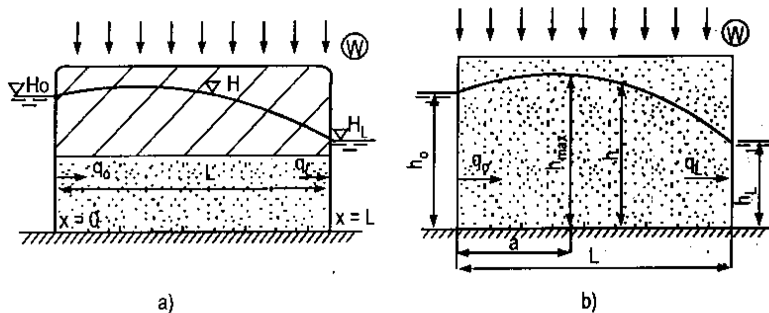
Hình VII-10. Dòng thấm đồng nhất có cường độ ngấm bổ sung ( W )
