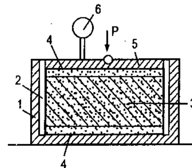
Hình V-6. Thiết bị nén đất trong phòng.
