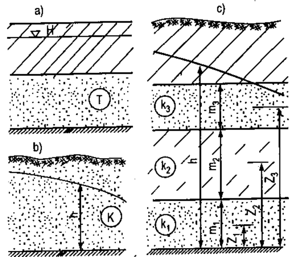
Hình VII-8. Các sơ đồ cấu tạo của dòng thấm phẳng đứng
