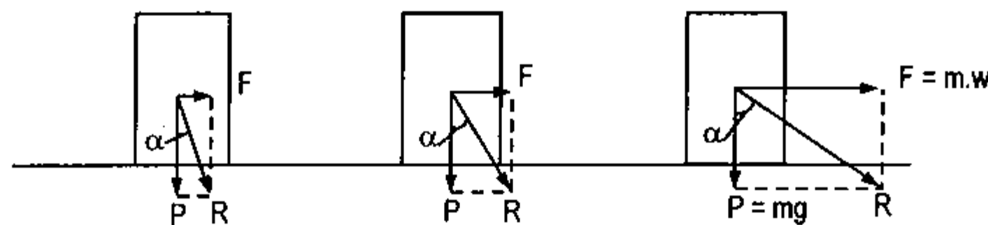
Hình VIII-40. Sơ đồ ổn định lật của công trình do động đất.
