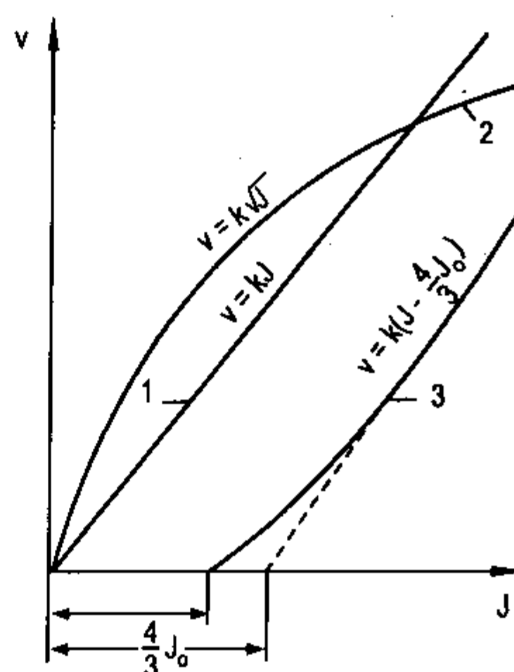
Hình VII-3. Biểu đồ quan hệ v = f(J) 1. Thấm tầng ; 2. Thấm rớt ; 3. Thấm dẻo nhớt
