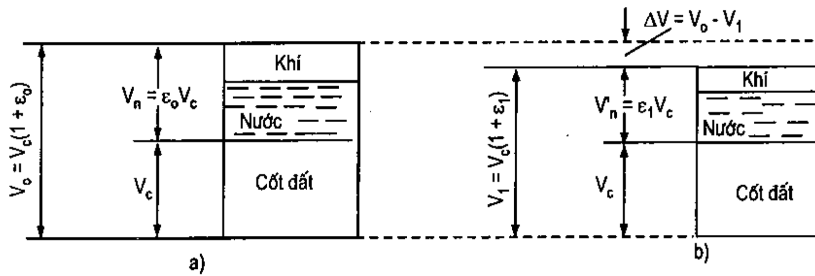
Hình V-7. Thay đổi thể tích lỗ rỗng của mẫu đất khi nén
