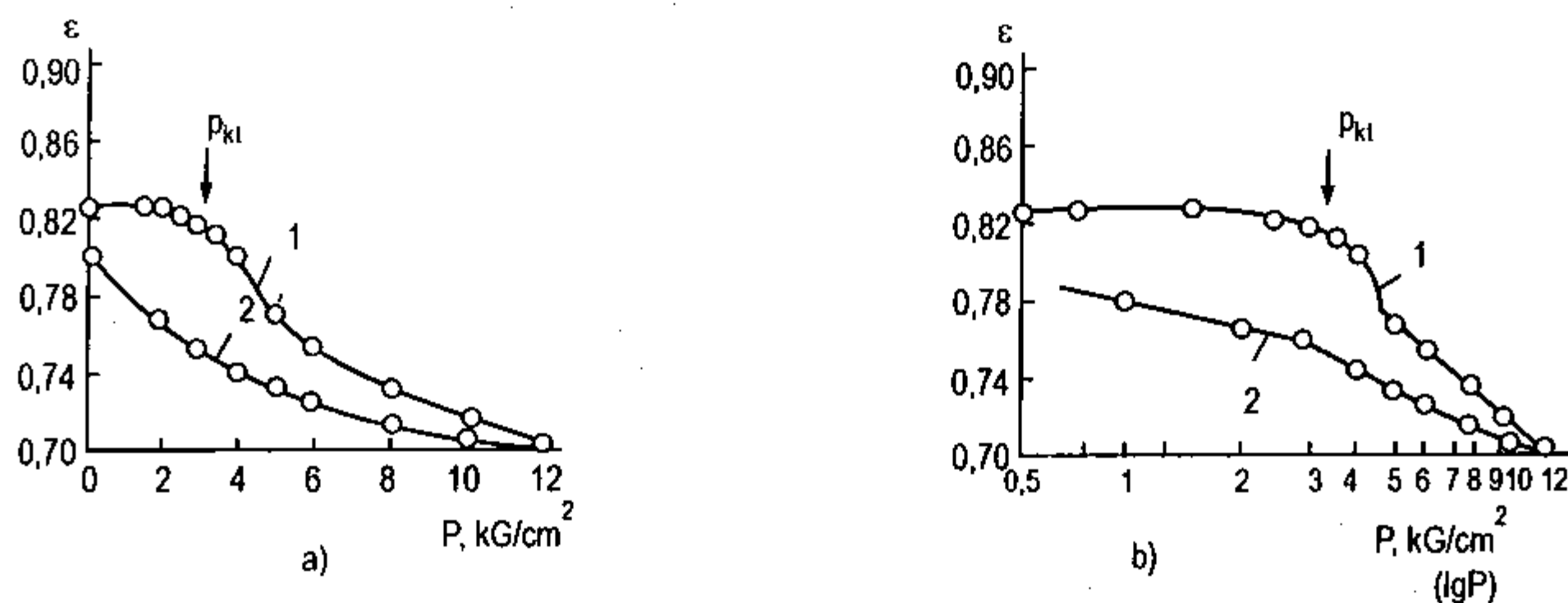
Hình V- 8. Đường cong nén
