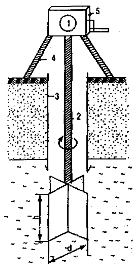
Hình IX-12. Sơ đồ thí nghiệm cắt quay
