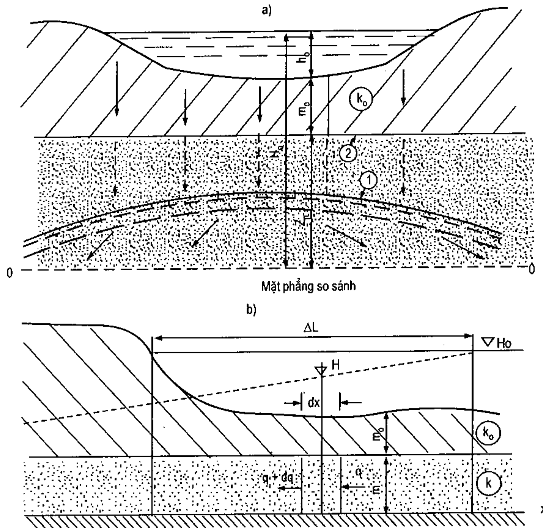
Hình VII-12. Sơ đồ dòng thấm dưới đáy hồ
