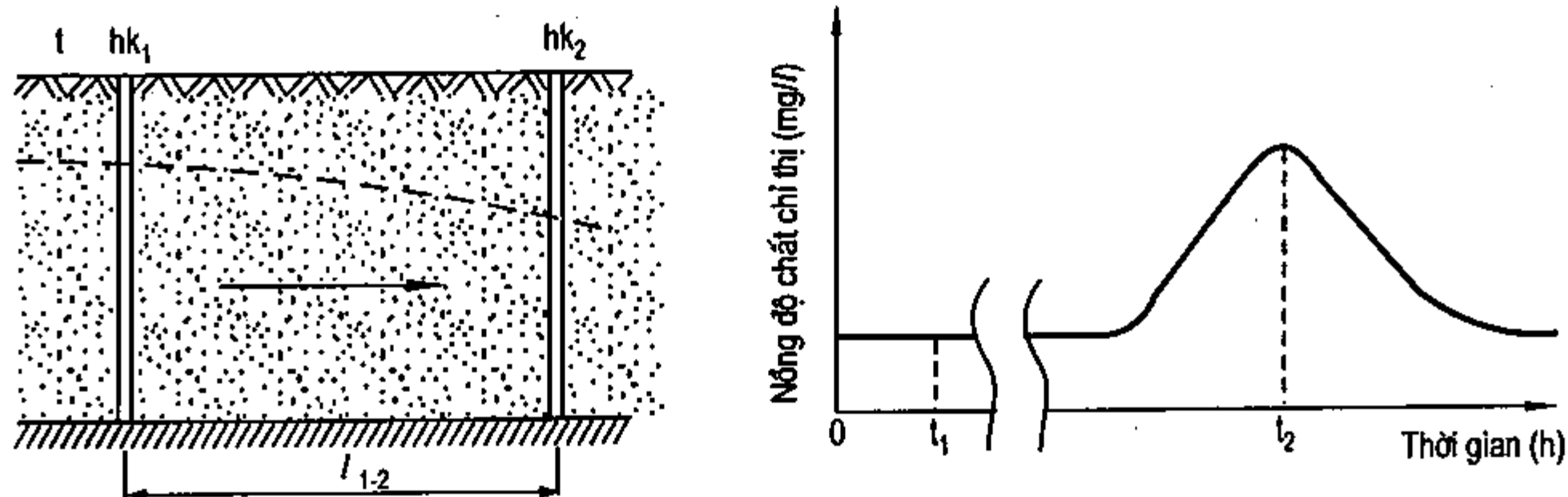
Hình VI-4. Sơ đồ xác định tốc độ chuyển động của nước dưới đất theo mặt cắt dọc lưu tuyến (hình trái) ; biểu đồ theo dõi chất chỉ thị ở hố khoan (hình phải)
