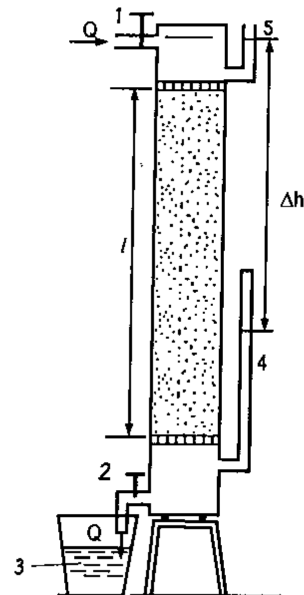
Hình VII-2. Dụng cụ thấm của Đacxi.
