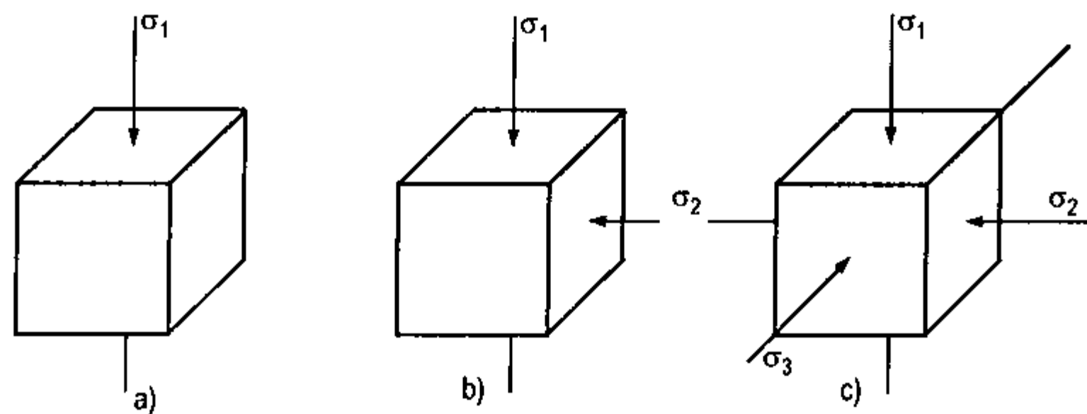
Hình V-1. Các trạng thái ứng suất trong đất đá
