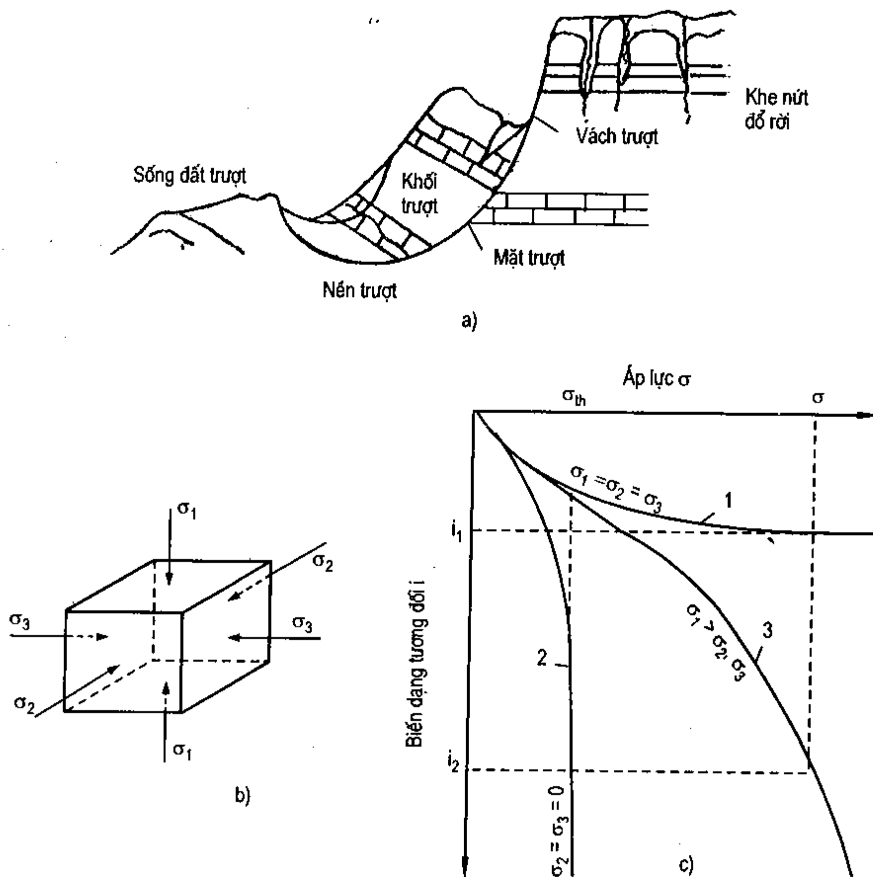
Hình VIII-26. Hiện tượng trượt đất.
