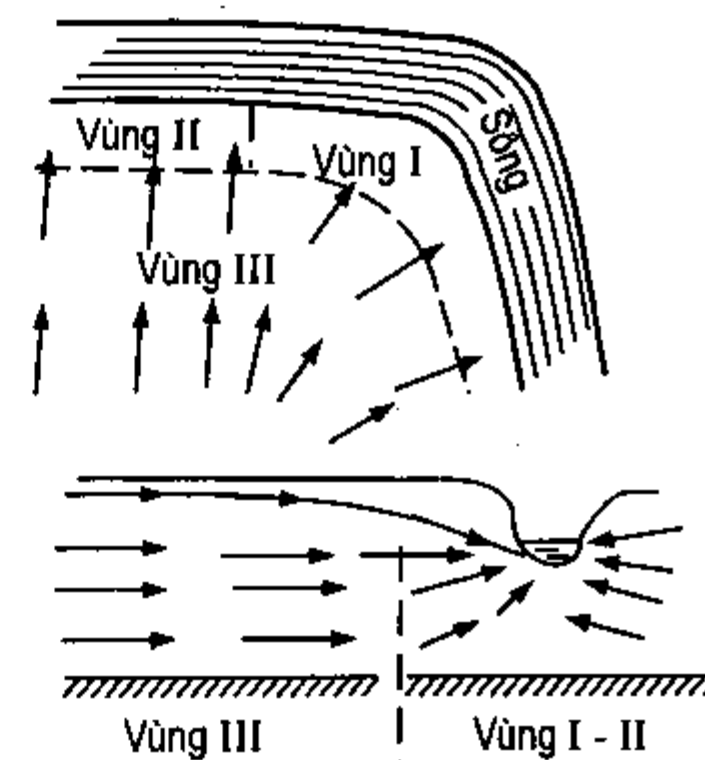
Hình VII-5. Sơ đồ các dạng dòng thấm a) Mặt bằng ; b) Mặt cắt
