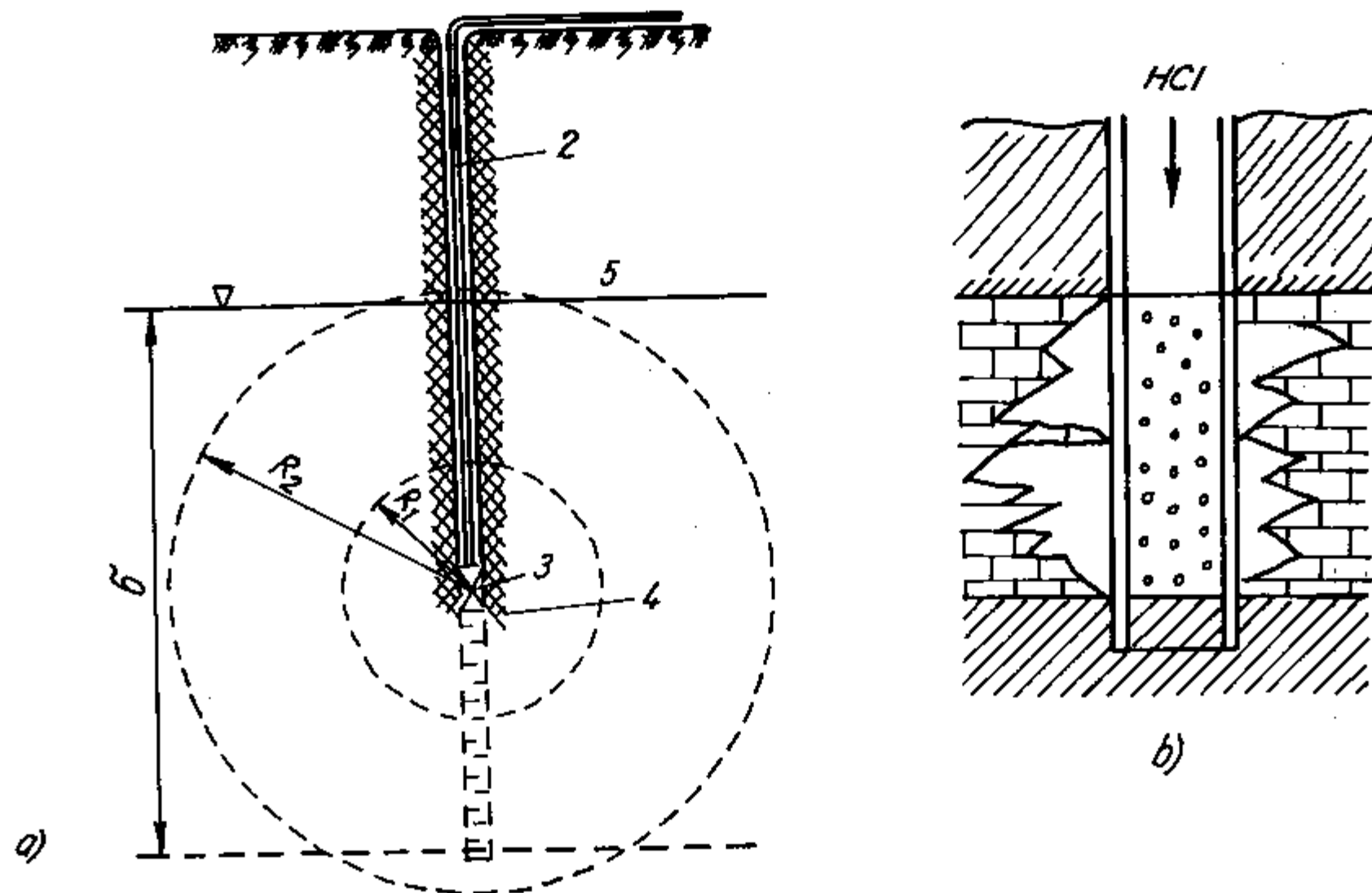
Hình X-1. Sơ đồ mở rộng khe nứt của đá ở gần hố khoan
