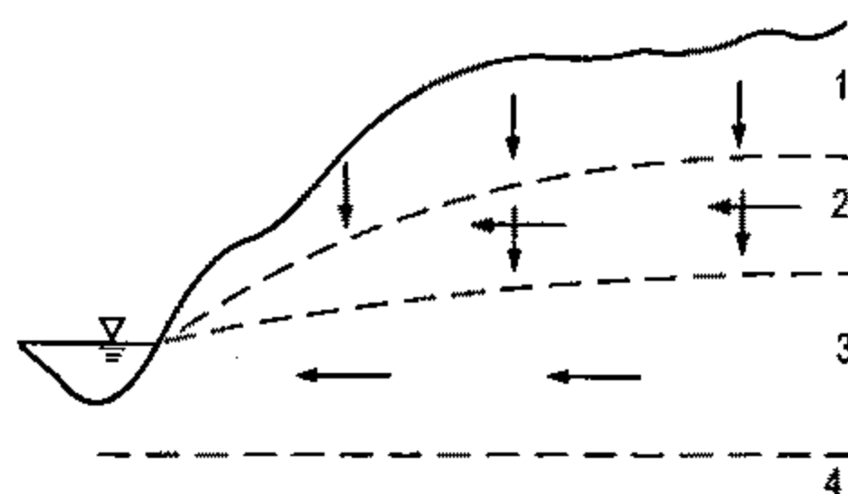
Hình VIII-24. Các đới karst
