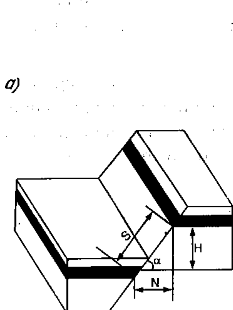
Hình II-3. Đứt gãy
