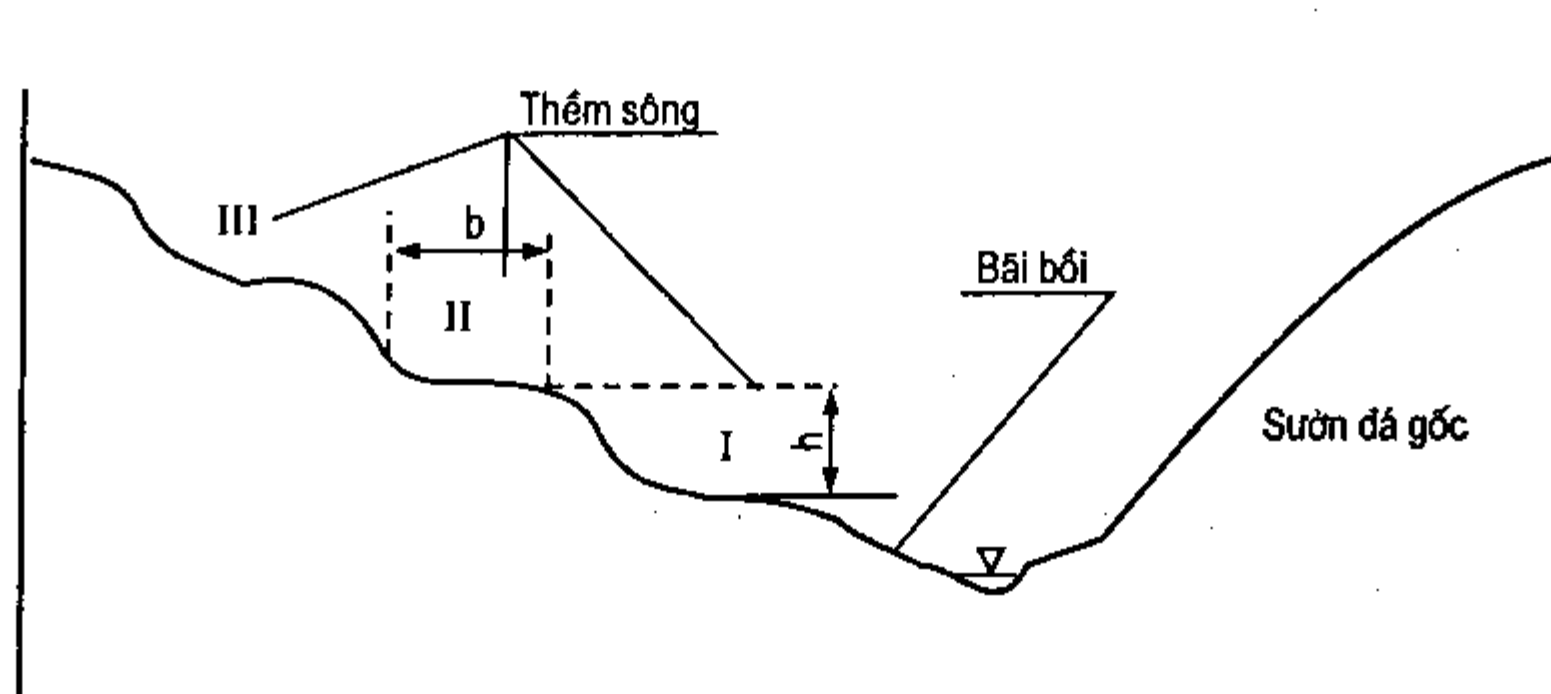
Hình VIII-5. Cấu tạo của lũng sông b- Bề rộng thêm ; h - Chiều cao thêm.
