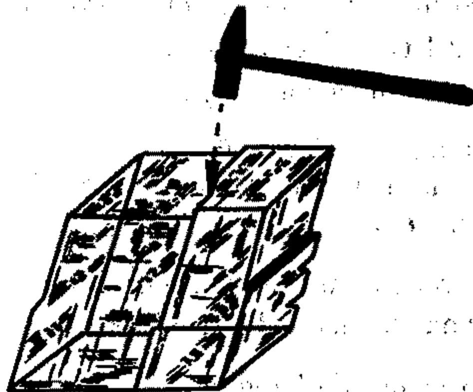
Hình I-2. Tính dễ tách hoàn toàn của canxit
