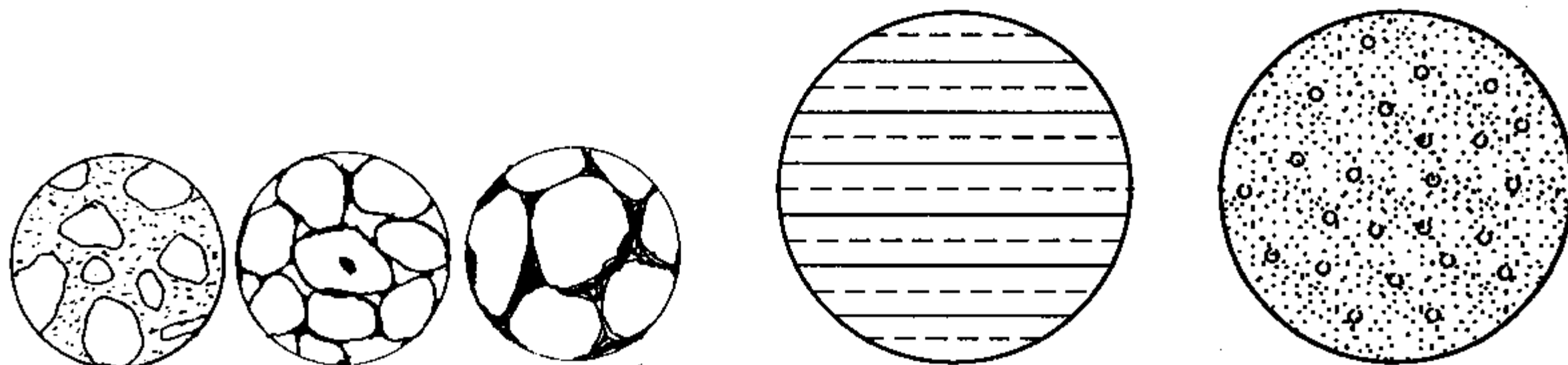
a) b) Hình I-15. Cấu tạo của đá trầm tích a) Cấu tạo lớp ; b) Cấu tạo khối.
