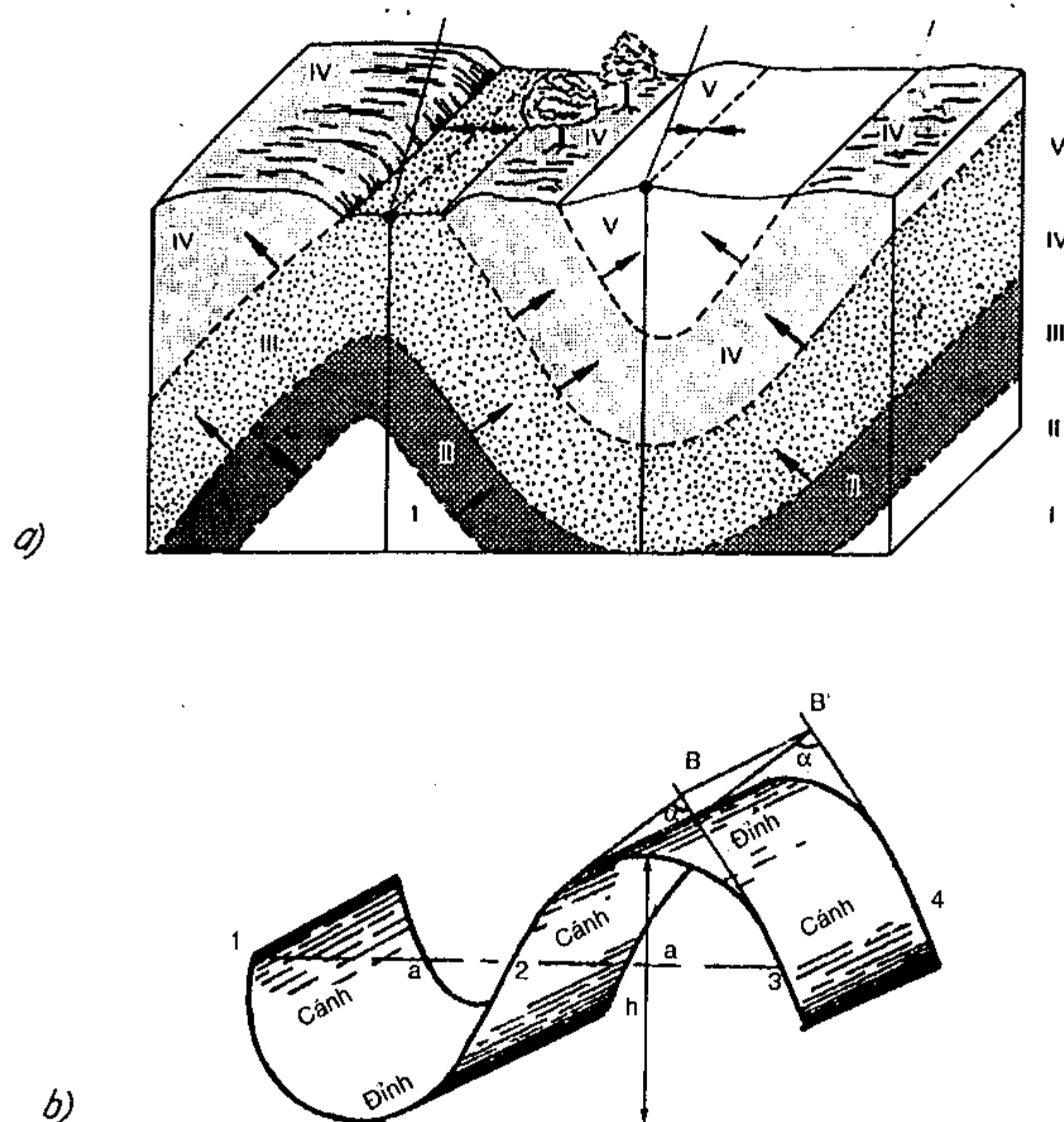
Hình II-2. Sơ đồ cấu tạo nếp uốn
