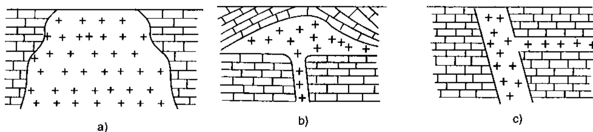
Hình I-5. Dạng thể nằm của đá xâm nhập.
