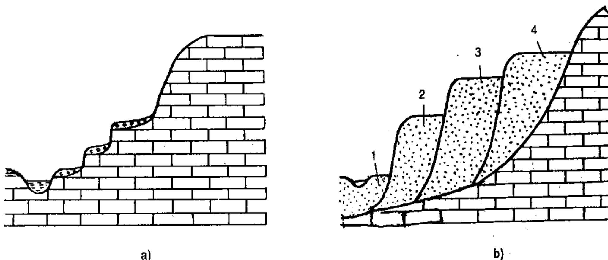
Hình VIII-6. Các loại thêm sông a) Thêm xâm thực ; b) Thêm tích tụ ; 1. Bãi bồi ; 2,3,4. Thêm sông .
