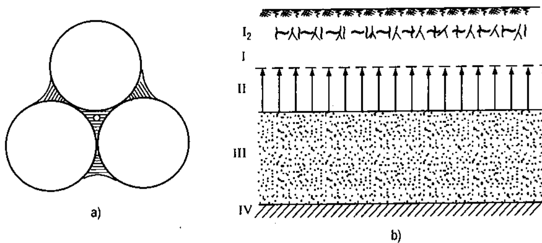
Hình IV-1. Các loại nước mao dẫn
