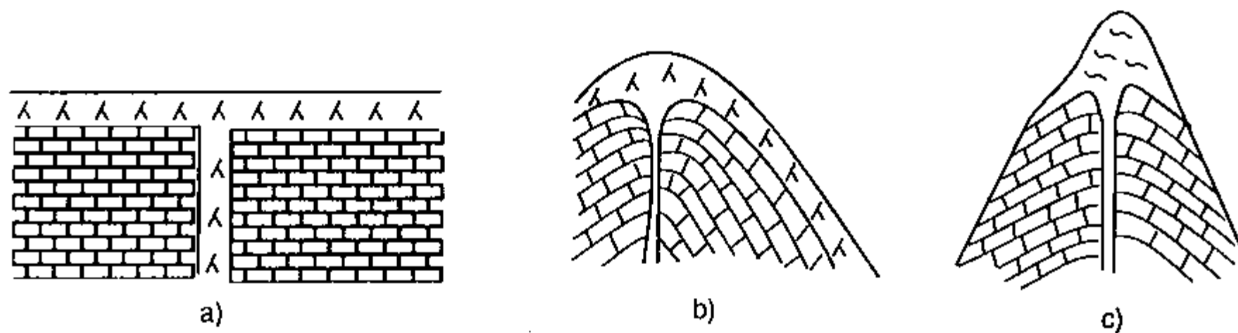
Hình I-6. Dạng thể nằm của đá phun trào
