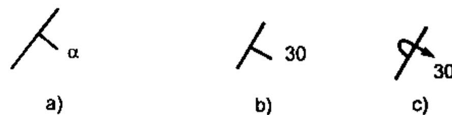
Hình I-11. Biểu thị các yếu tố thể nằm tầng đá trên bản đồ địa chất
