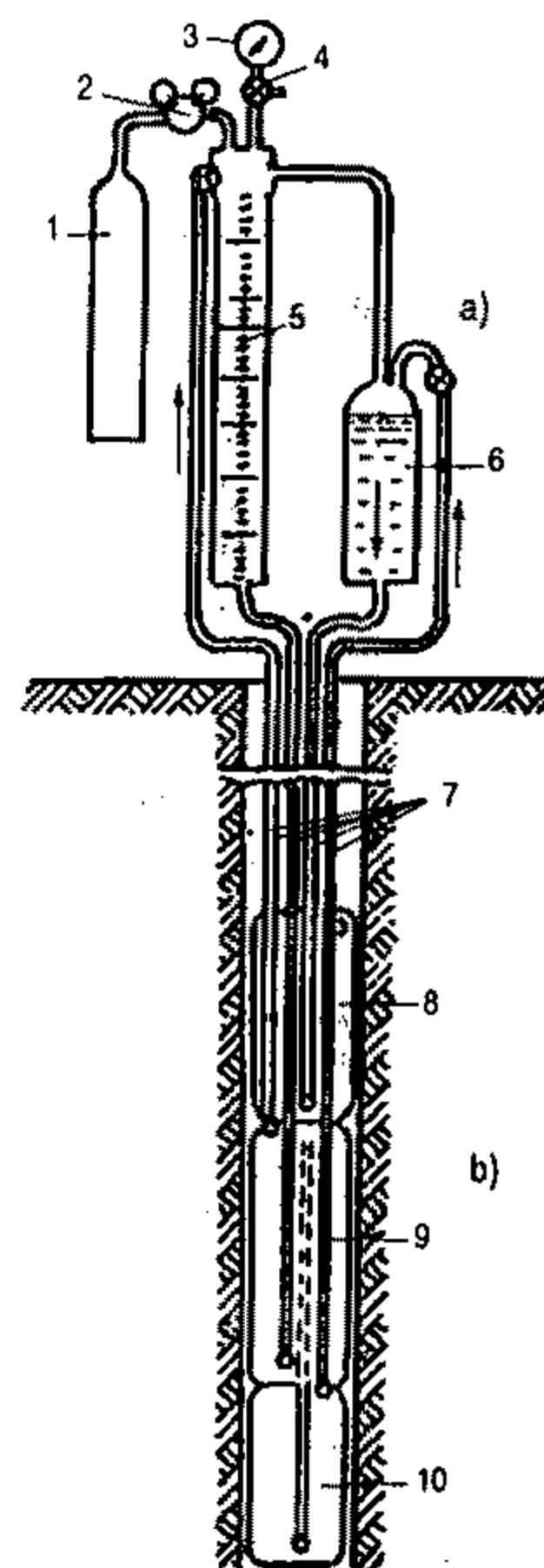
Hình IX-10. Sơ đồ máy ép
