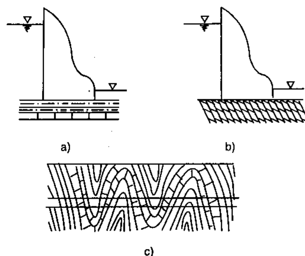
Hình II-6. Ảnh hưởng của biến vị kiến tạo đến xây dựng
