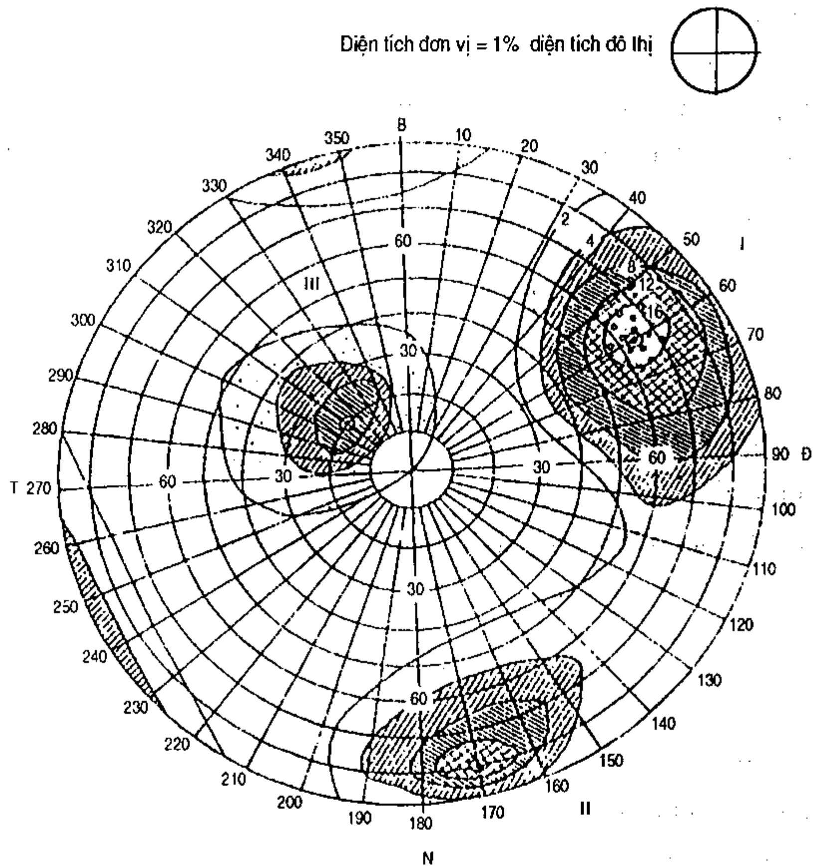
Hình IV-3. Đồ thị vòng tròn khe nứt, sau khi vẽ đường đồng mức đã nổi lên ba nhóm khe nứt. Các nhóm chính I và II gần vuông góc với nhau ; nhóm phụ III gần nằm ngang.
