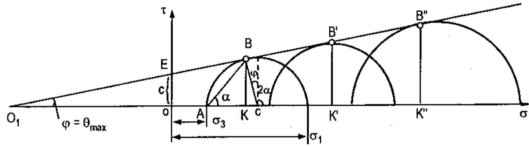
Hình V-5. Dùng vòng tròn Mor xác định trạng thái ứng suất của đất đá
