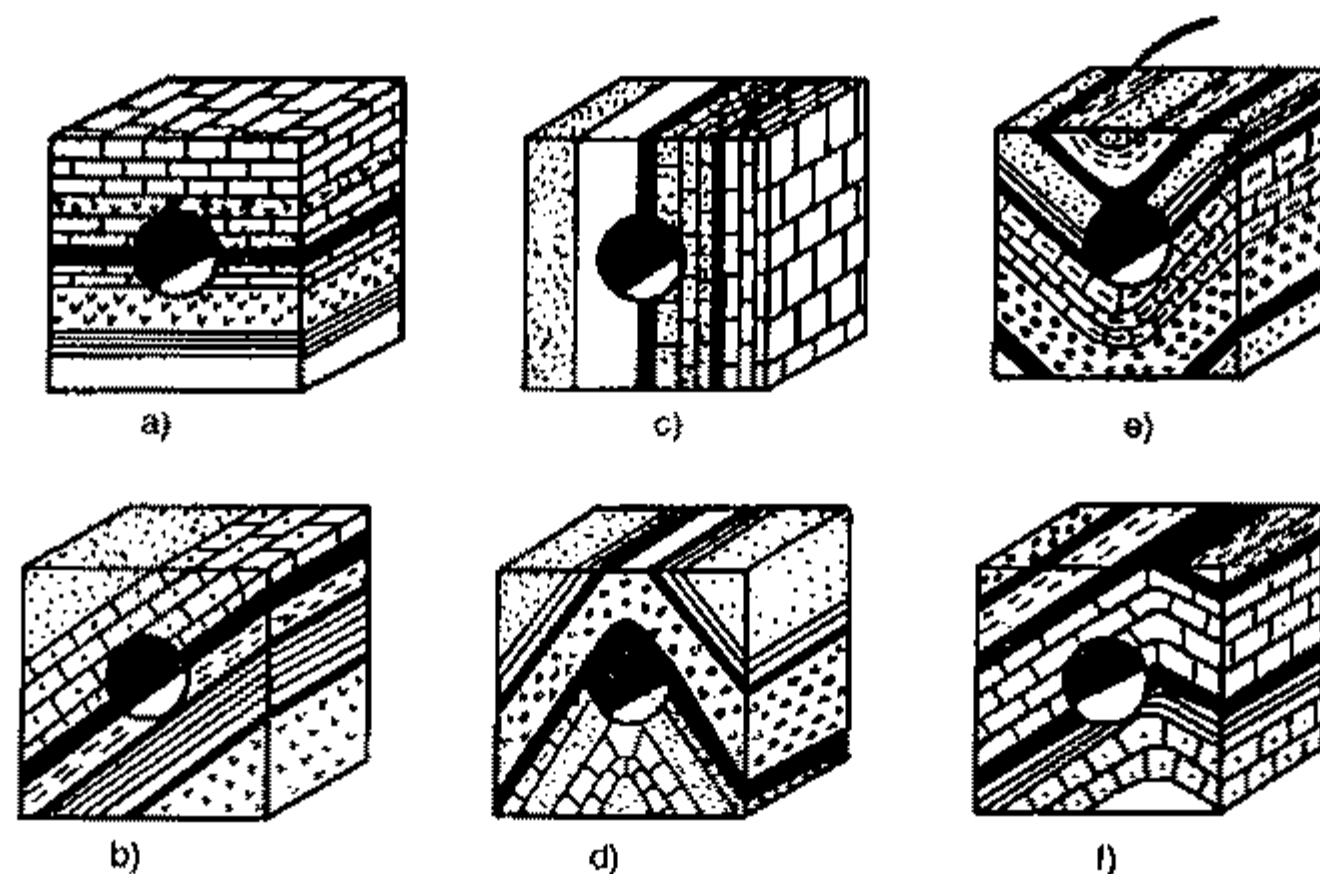
Hình II-10. Đường hầm song song với đường phương tầng đá.
