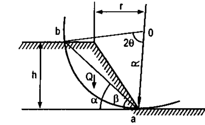
Hình VIII-32. Xác định độ ổn định của mái dốc theo cung trượt tới hạn.
