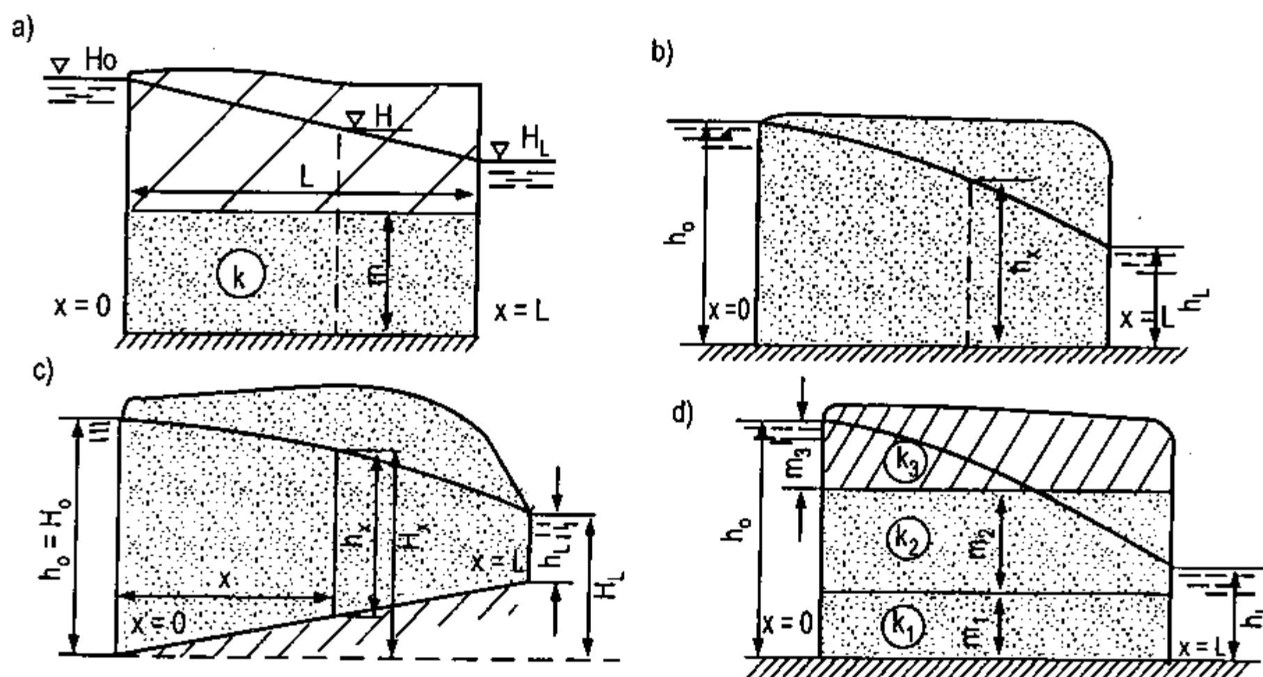
Hình VII-9. Sơ đồ các dạng thấm phẳng đứng
