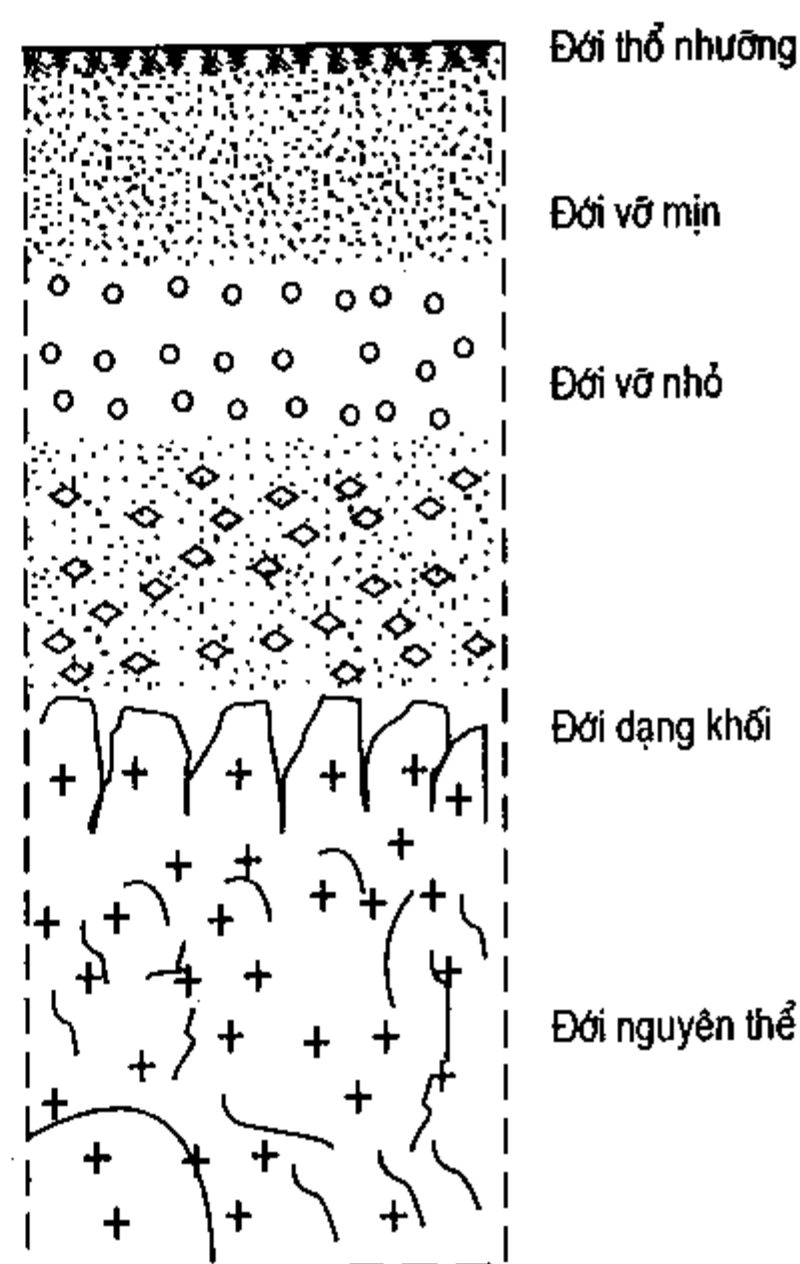
Hình VIII-1. Các đới phong hóa
