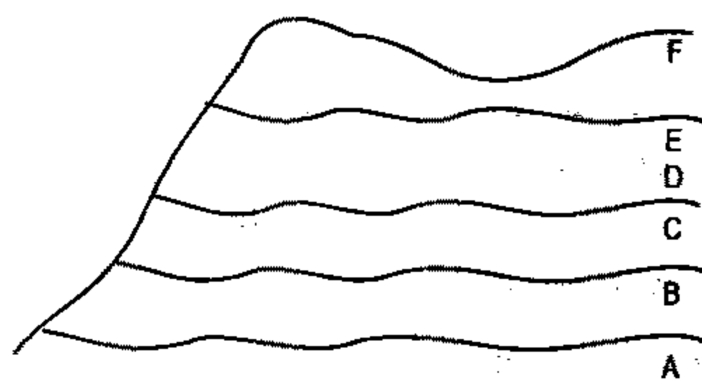
Hình VIII-3. Sơ đồ mặt cắt laterit (theo Phốc)
