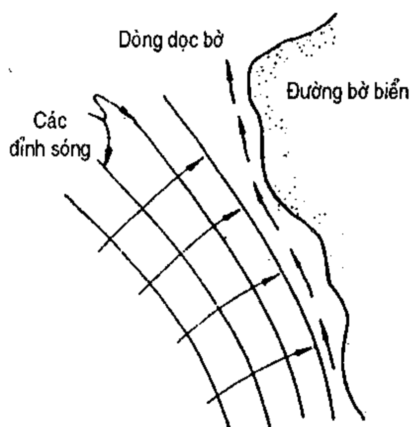
Hình VIII-17. Dòng dọc bờ liên quan với các sóng tiến xiên góc vào bờ
