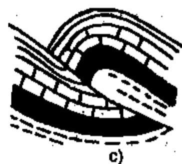
Hình II-4 . Các loại đứt gãy
