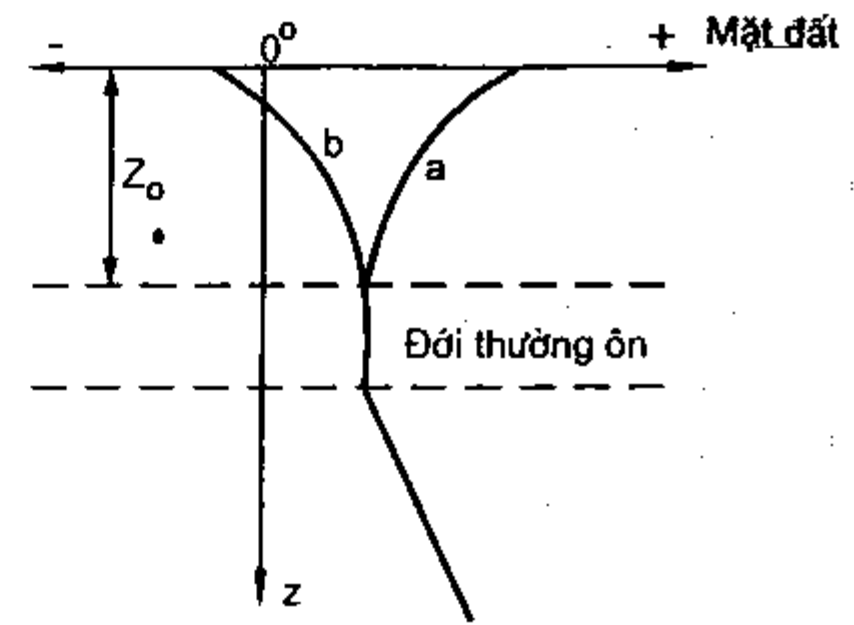
Hình I-1. Sơ đồ nhiệt theo độ sâu của vỏ quả đất
