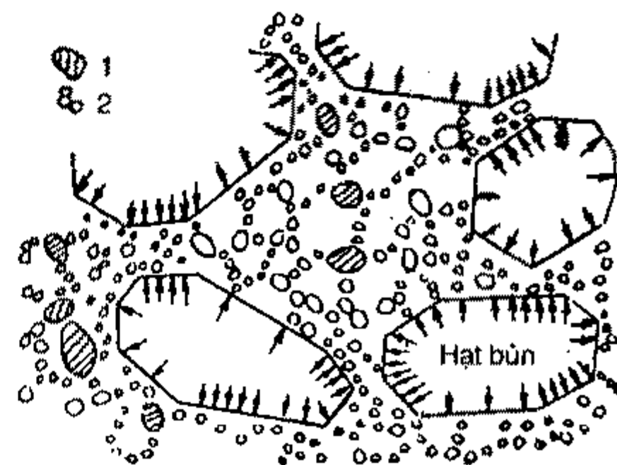
Hình I-13. Kiến trúc của đất sét biển 1. Hạt sét ; 2. Hạt keo.
