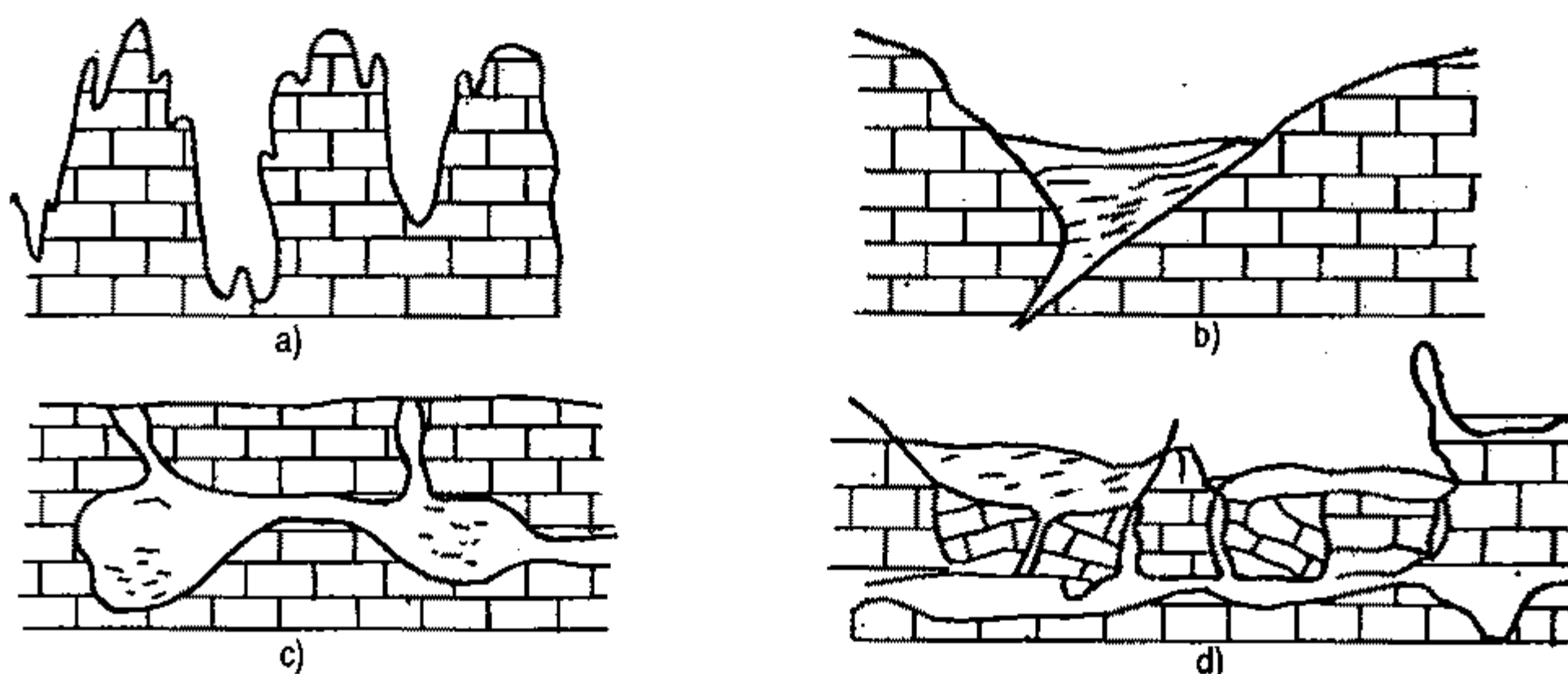
Hình VIII-23. Các hình thái karst
