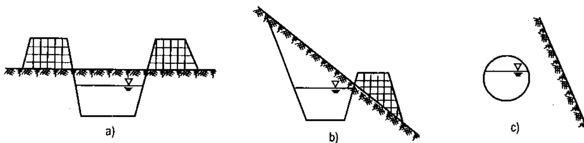
Hình III-7. Các hình thức kênh do địa mạo
