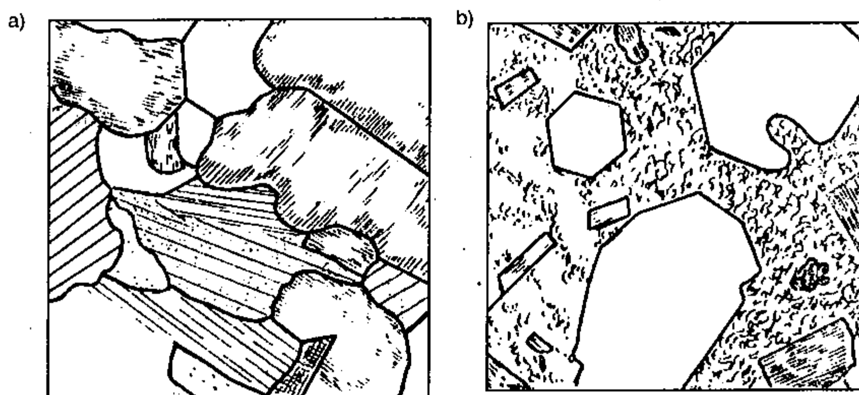
Hình I-8. Kiến trúc của đá macma (phóng đại 12 lần)
