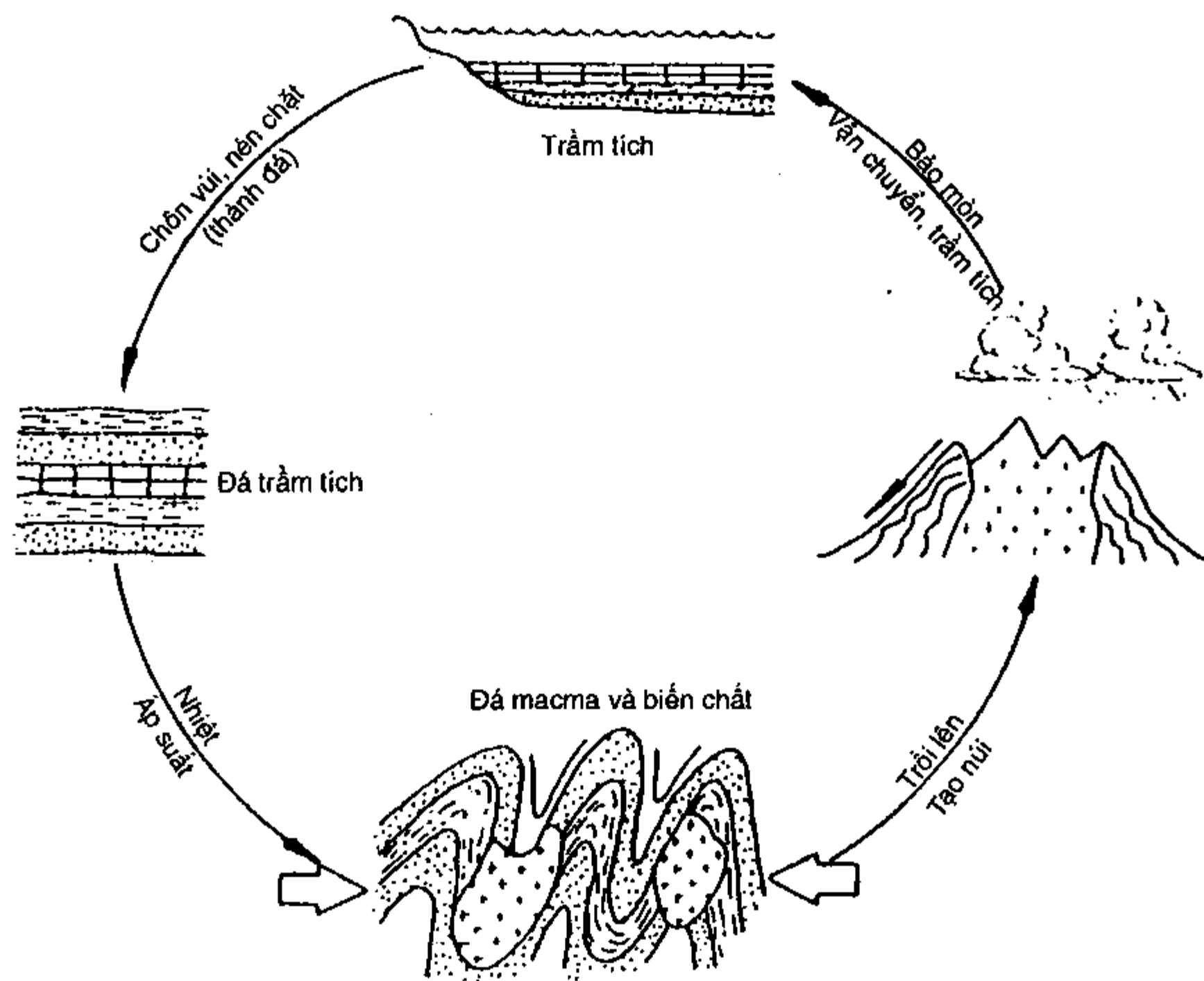
Hình I-19. Chu kỳ biến đổi của đất đá theo sự chuyển hoá của địa chất
