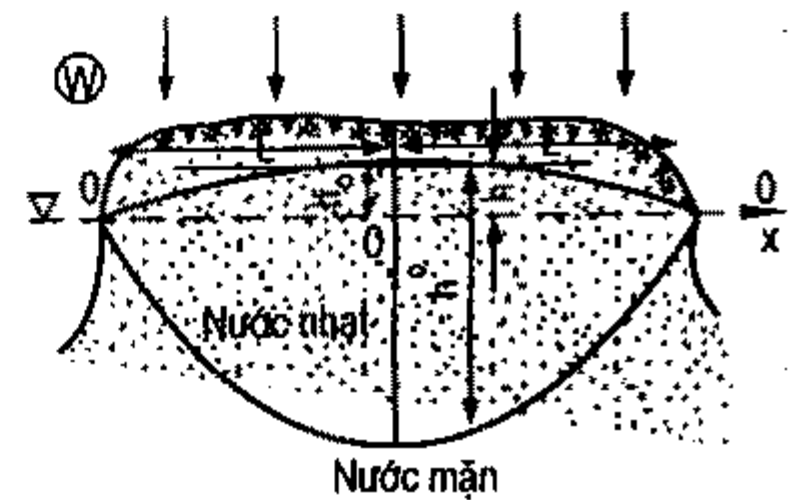
Hình VII-11. Thấu kính nước nhạt trên đảo.
