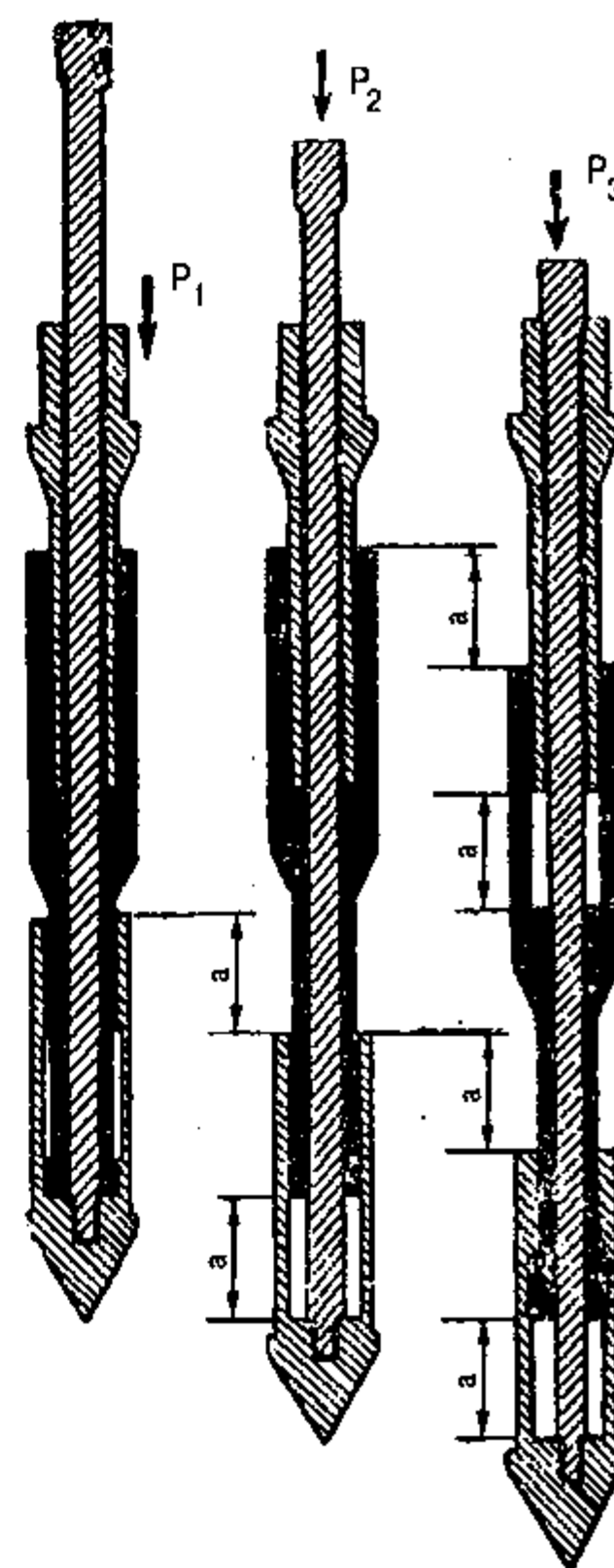
Hình IX-13. Sơ đồ thí nghiệm xuyên tại hiện trường
