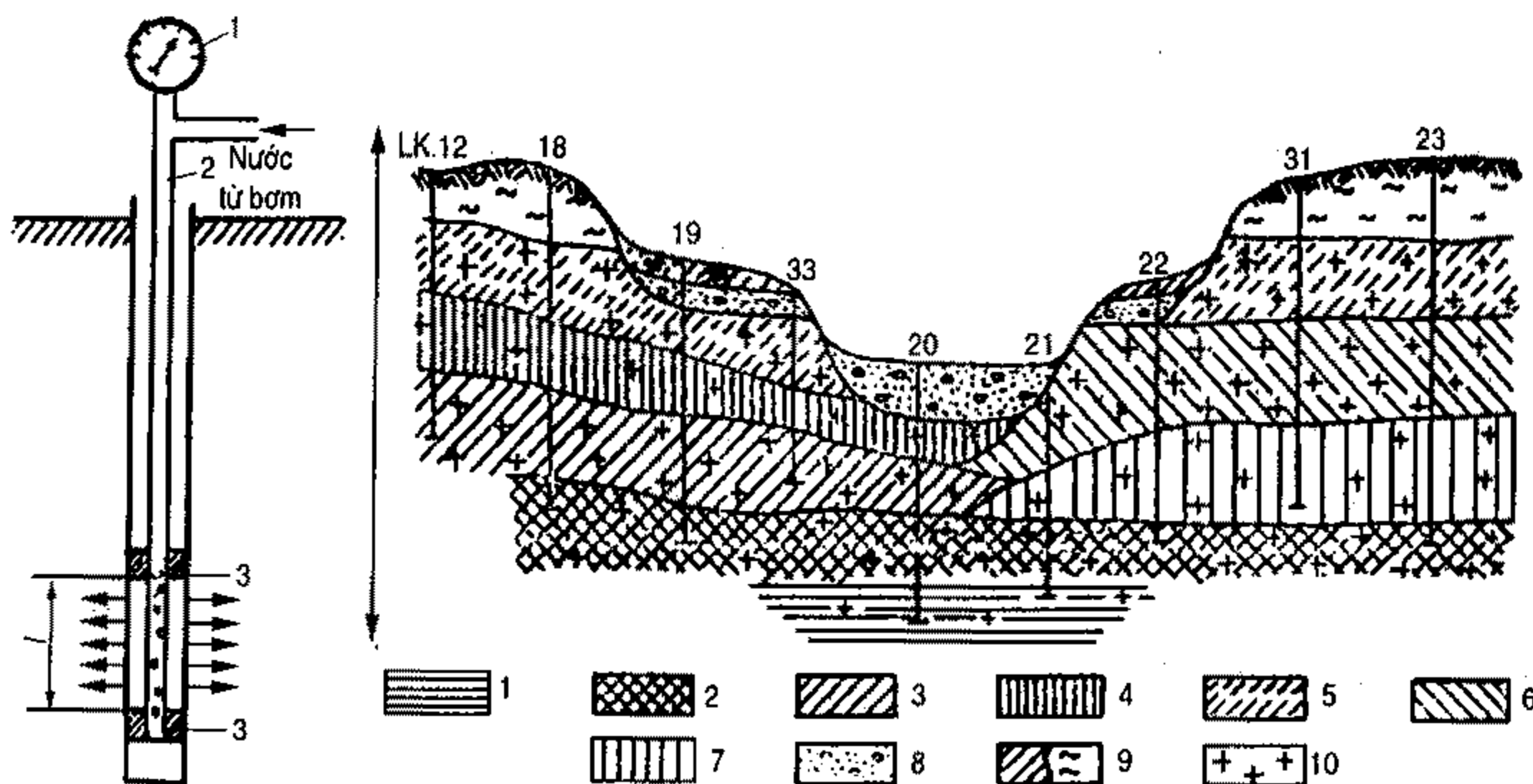
Hình IX-7. Mặt cắt địa chất theo tuyến đập, kèm theo độ hấp thụ nước đơn vị, l/ph 1. < 0,01 ; 2. 0,01 \div 0,05 ; 3. 0,05 \div 0,1 ; 4. 0,1 \div 0,5 ; 5. 0,5 \div 1 ; 6. 1 \div 5 ; 7. 5 \div 15 ; 8. Các hoi tích cuội và cát; 9. Tàn tích loại sét; 10. Đá granit
